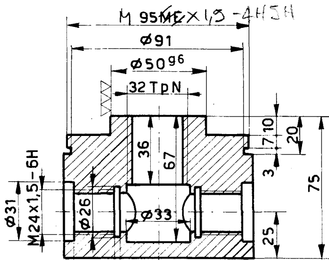
SEZ. A-A SCALA 1:2
